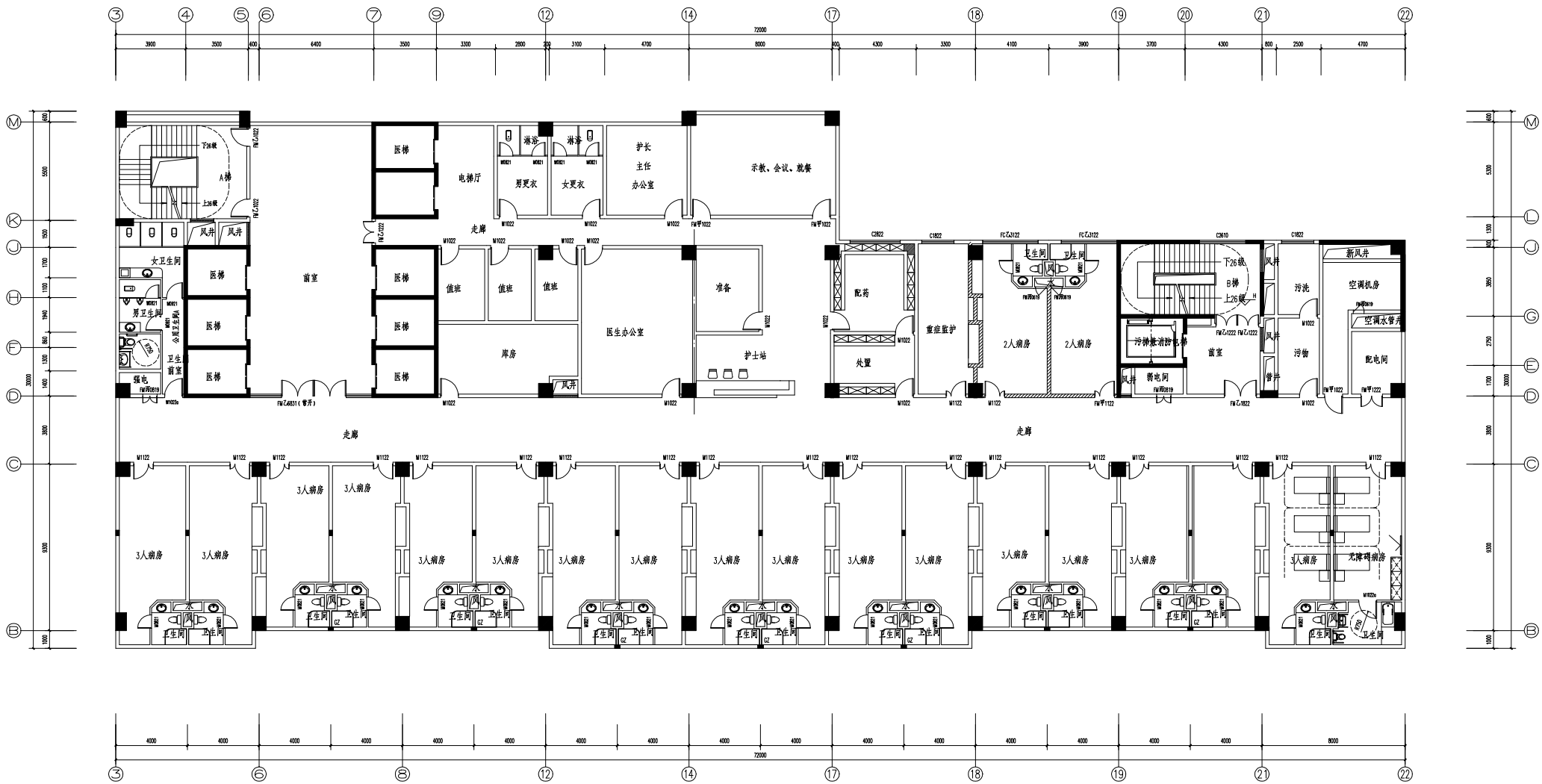
六至十三层平面图 1:100 本层建筑面积: 1885.22m²
